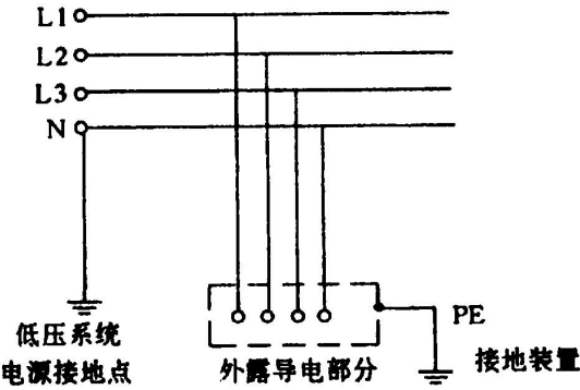
图 4 TT 系统
