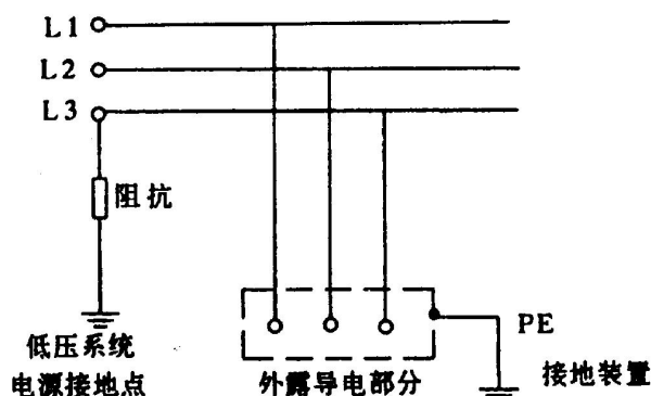
图 5 IT 系统
