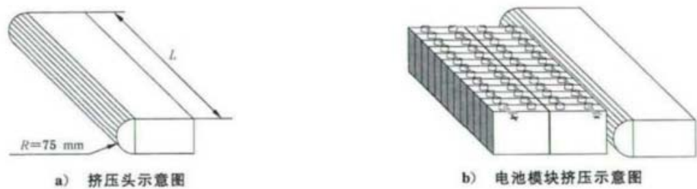
图 3 挤压头和电池模块挤压示意图
