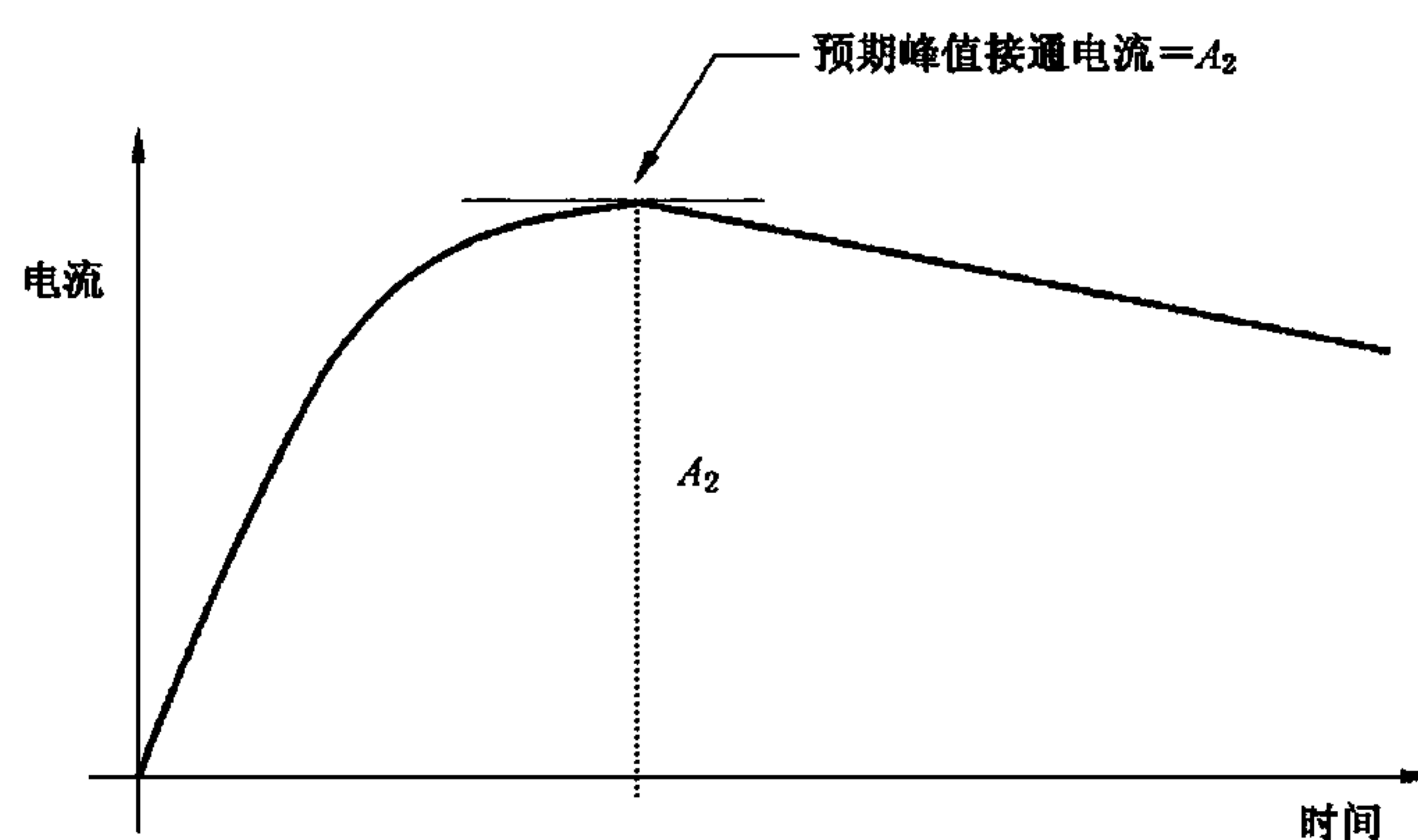
图 7b) 直流电流试验电路调整
