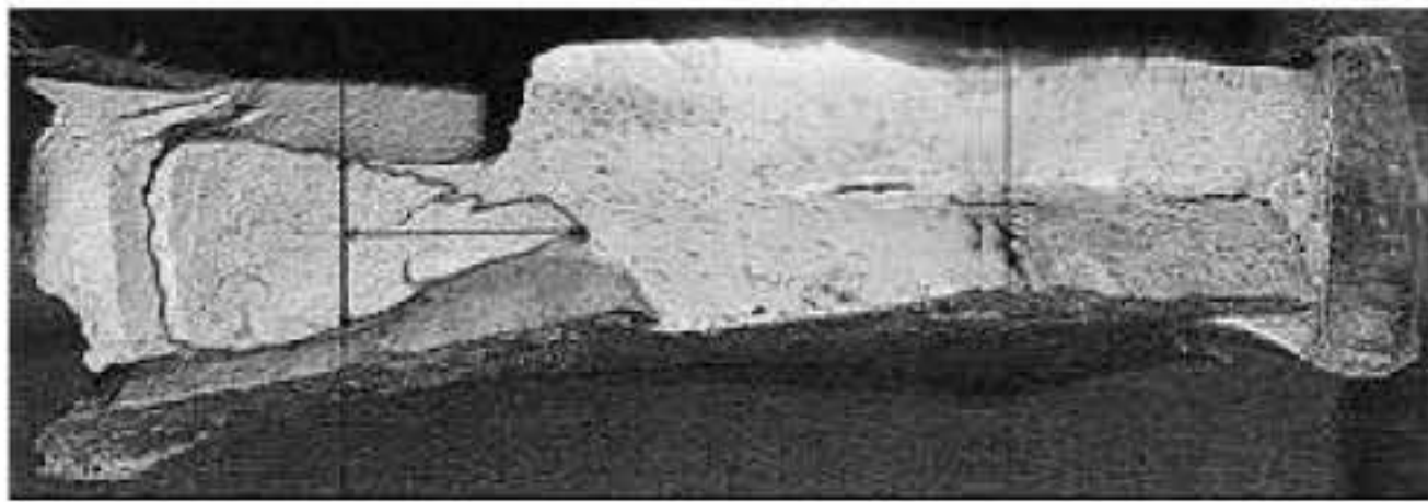
b) 第Ⅱ类异常断口
