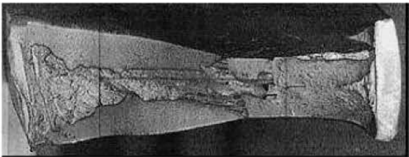
c) 第Ⅲ类异常断口
