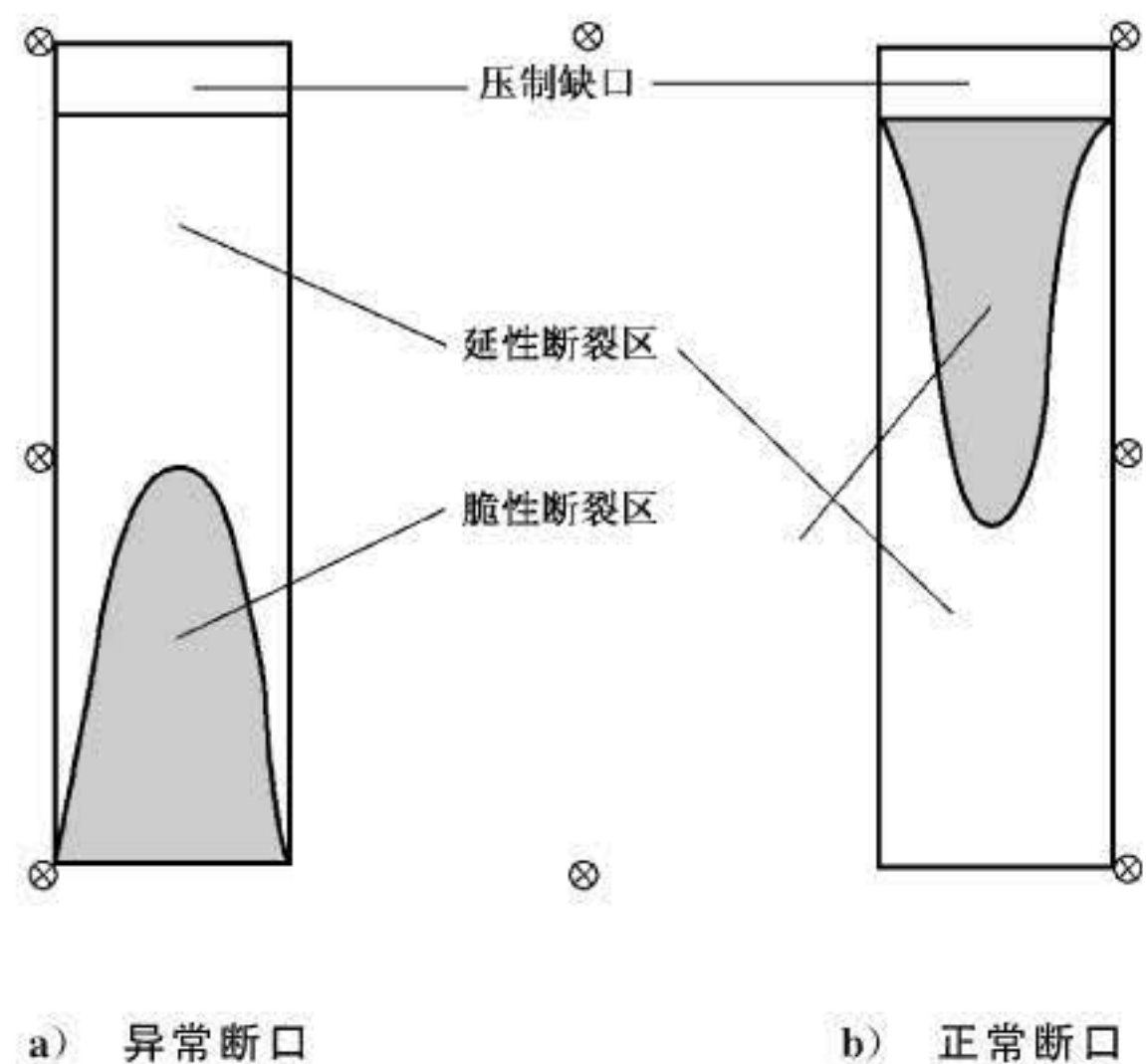
图 M.1 正常/异常典型断口示意图
