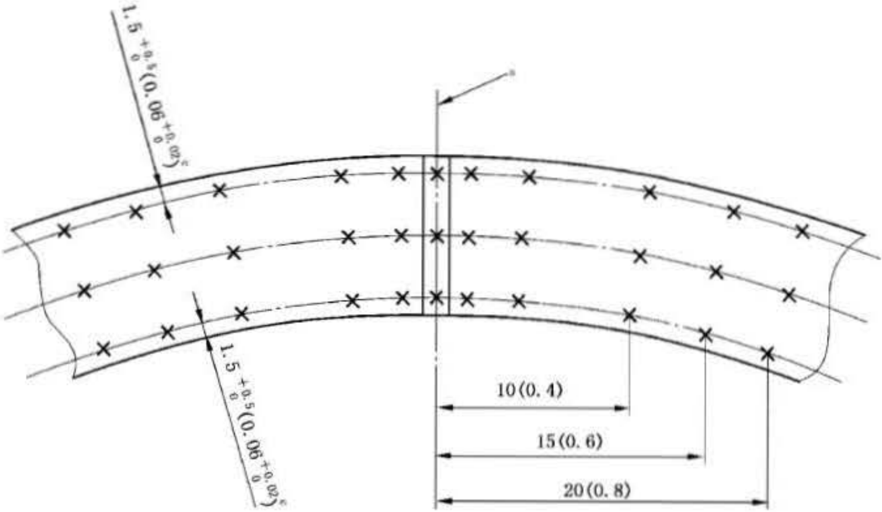
c) HFW 管
