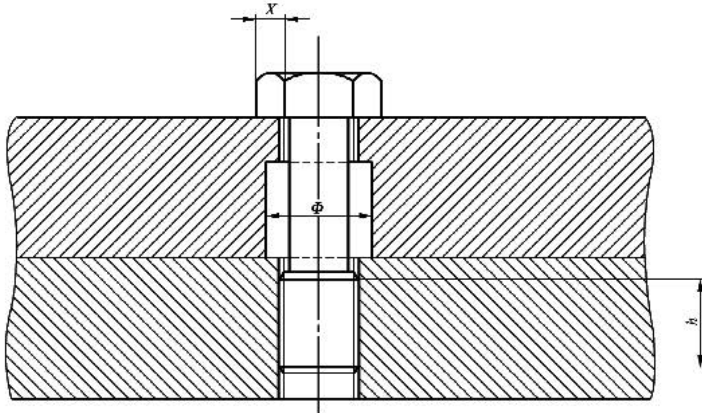
图 1 螺纹紧固件的公差和间隙
