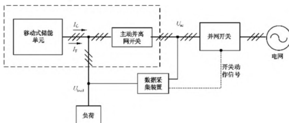
图3 并网切换试验回路示意图
