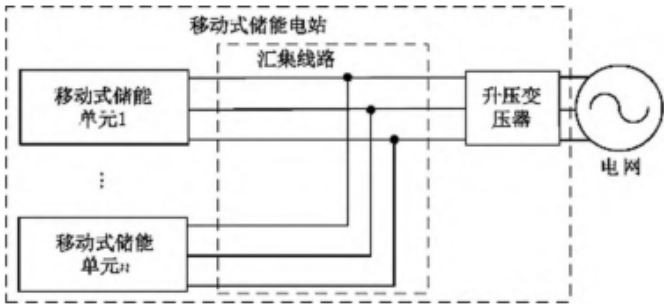
图 1 移动式储能电站架构图
