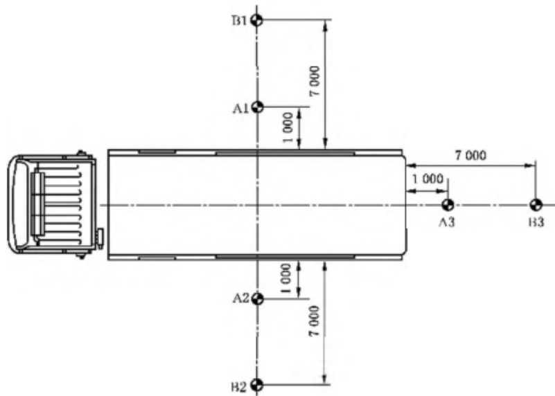
图4 噪声试验示意图
