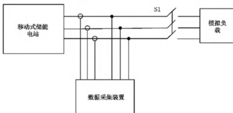
图6 离网性能试验连接图
