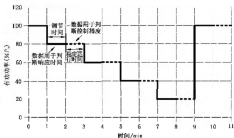
图5 有功功率控制曲线
