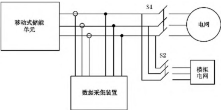
图 2 试验电路接线图
